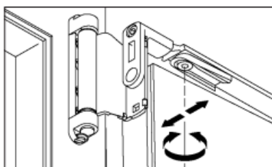
Nastavitev pritiska krila na okvir
